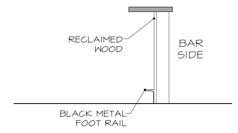
BAR DETAIL SCALE: 1/2"=1'-0"
