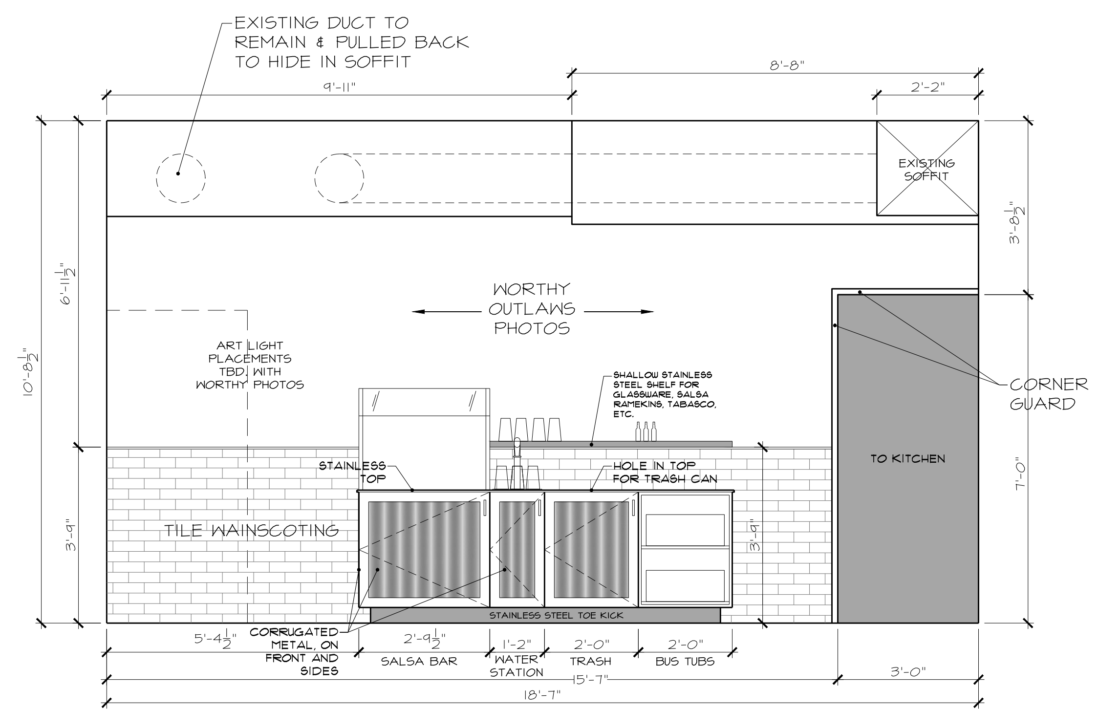
(E) TACO BAR SCALE: 3/8"=1'-0"
