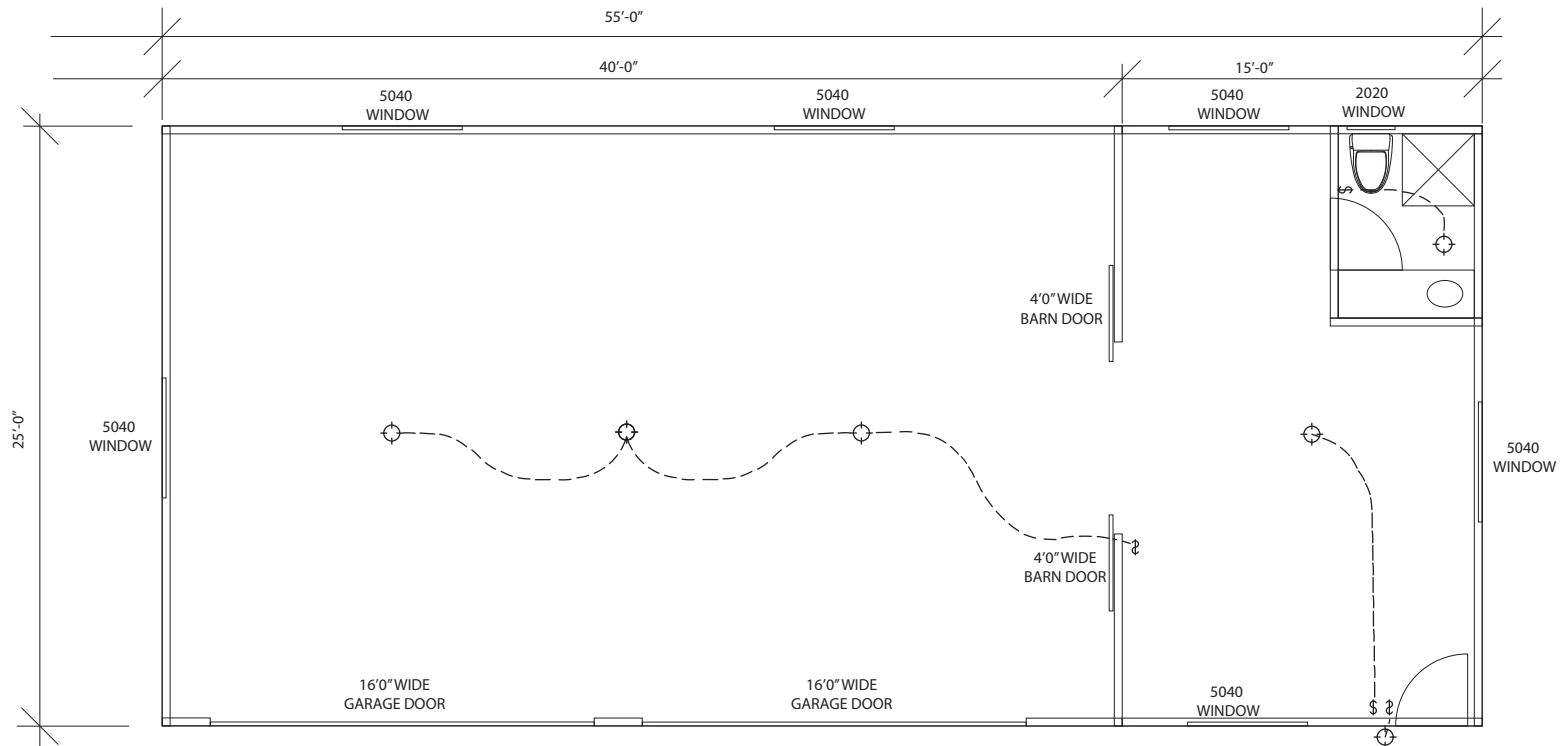
BARN FLOORPLAN SCALE: 1/8" = 1'
